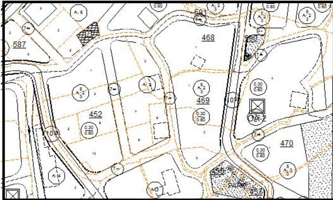
RESİM 2: Mevcut plan
